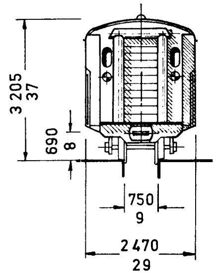
Wagenkastenlänge 14 540 mm 168 mm
